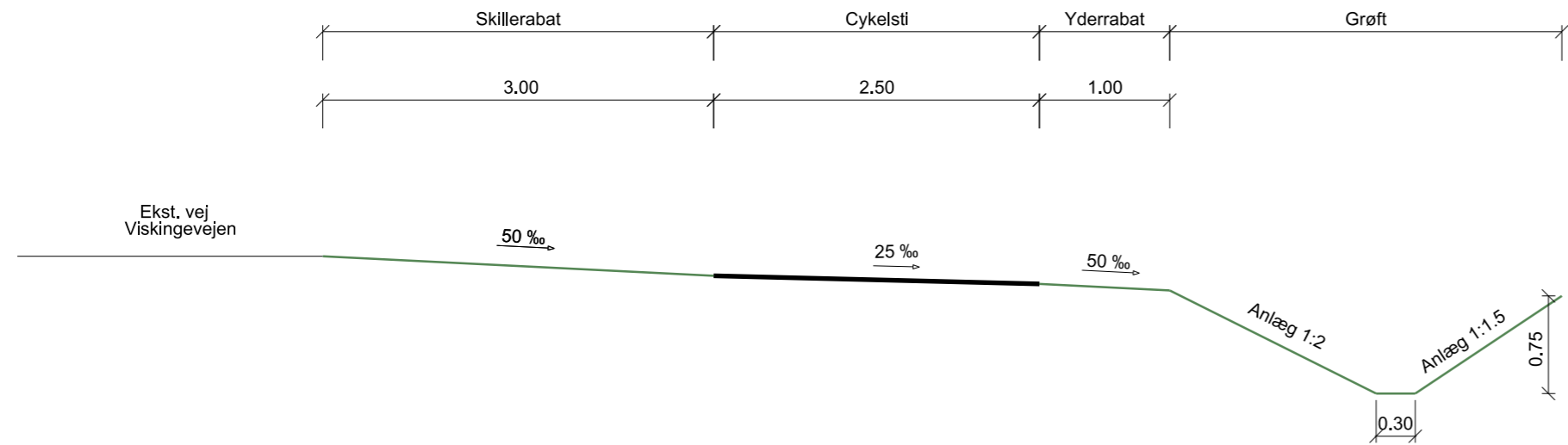
Principtværsnit - Dobbeltrettet cykelsti langs Viskingevejen
